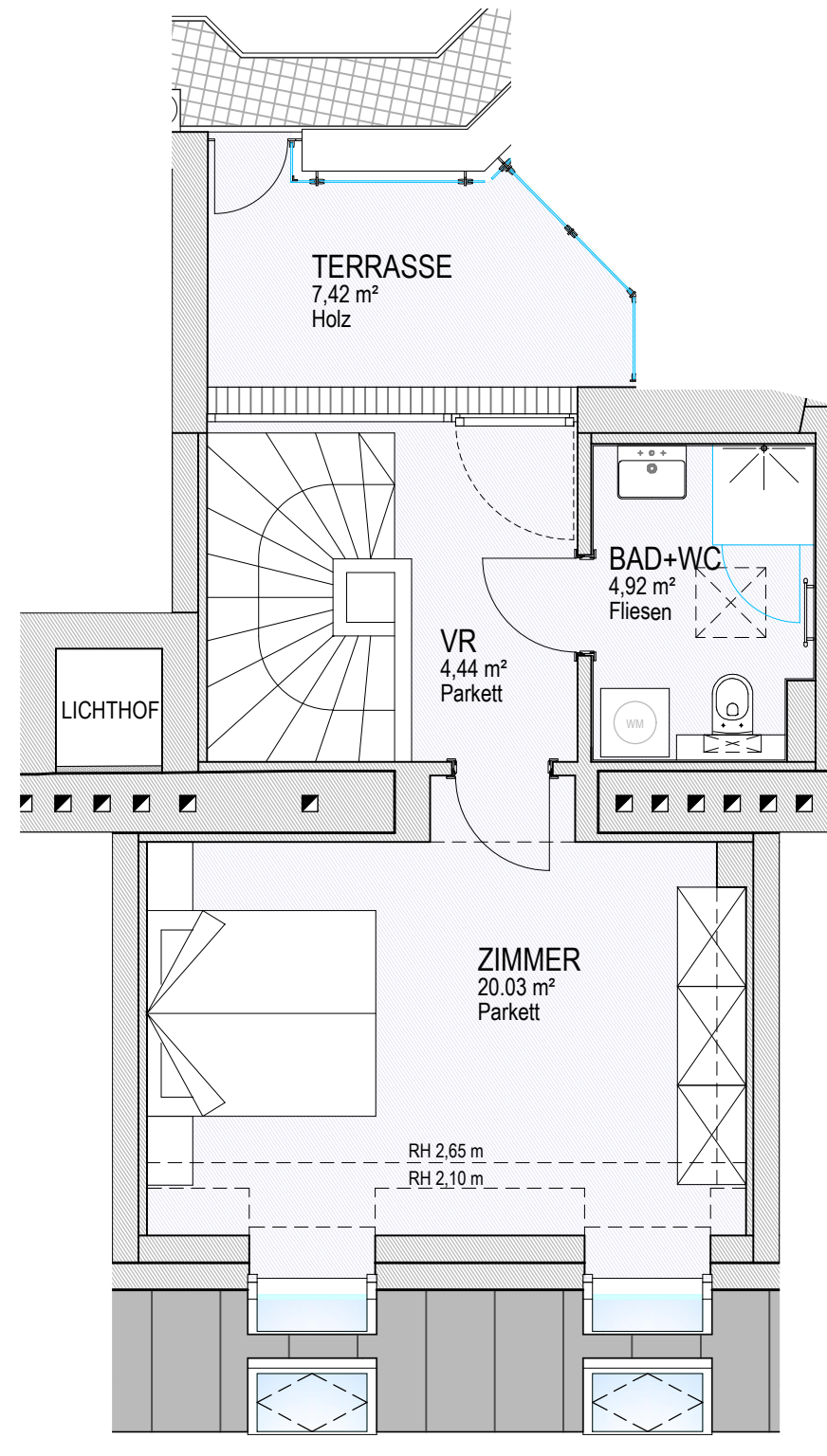
GRUNDRISS 2. DACHGESCHOSS
