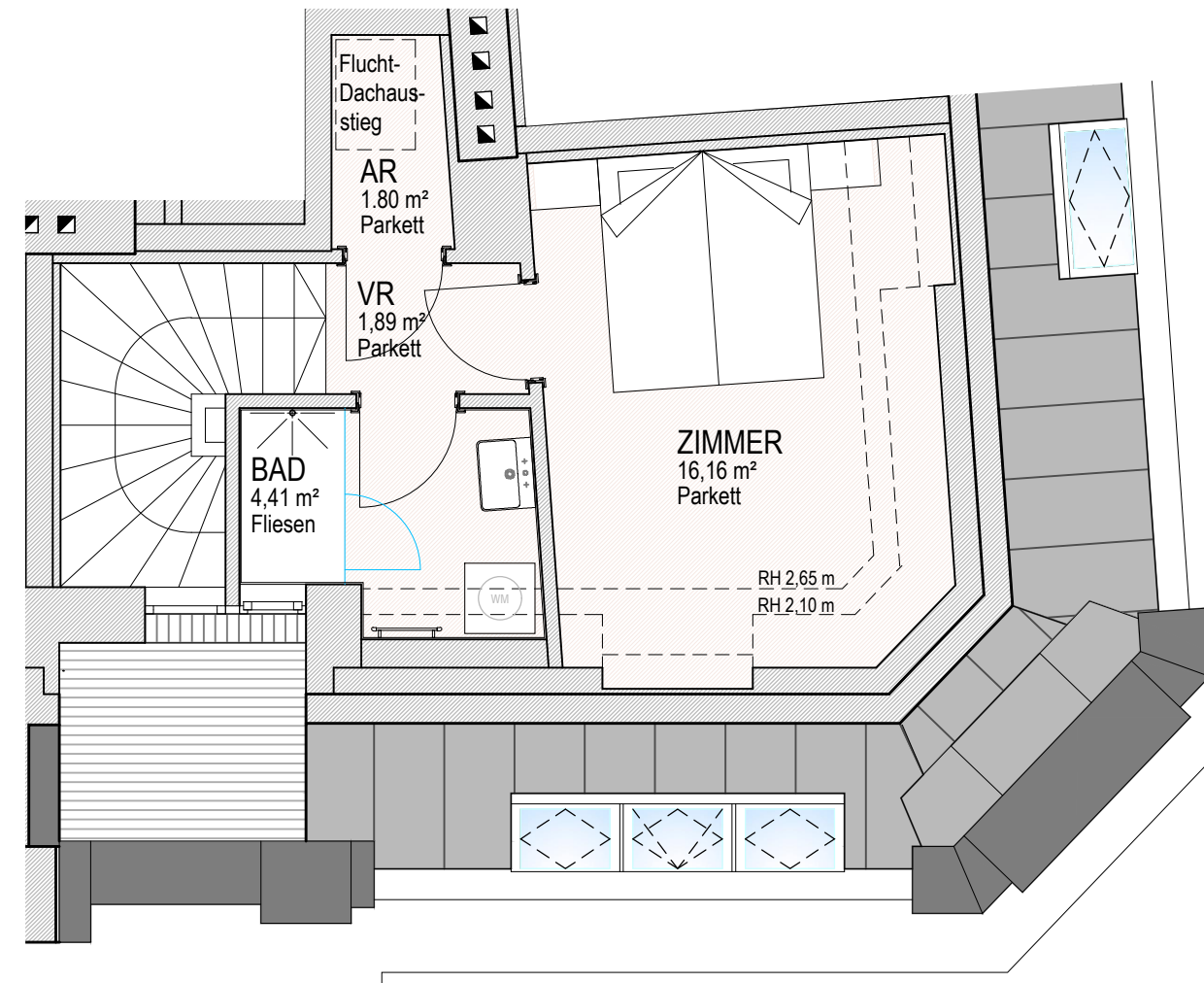
GRUNDRISS 2. DACHGESCHOSS
