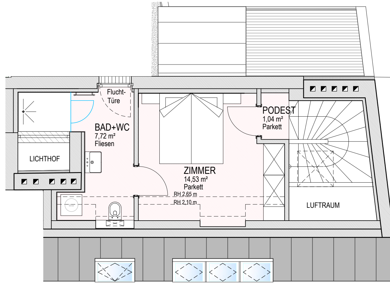
GRUNDRISS 2. DACHGESCHOSS
