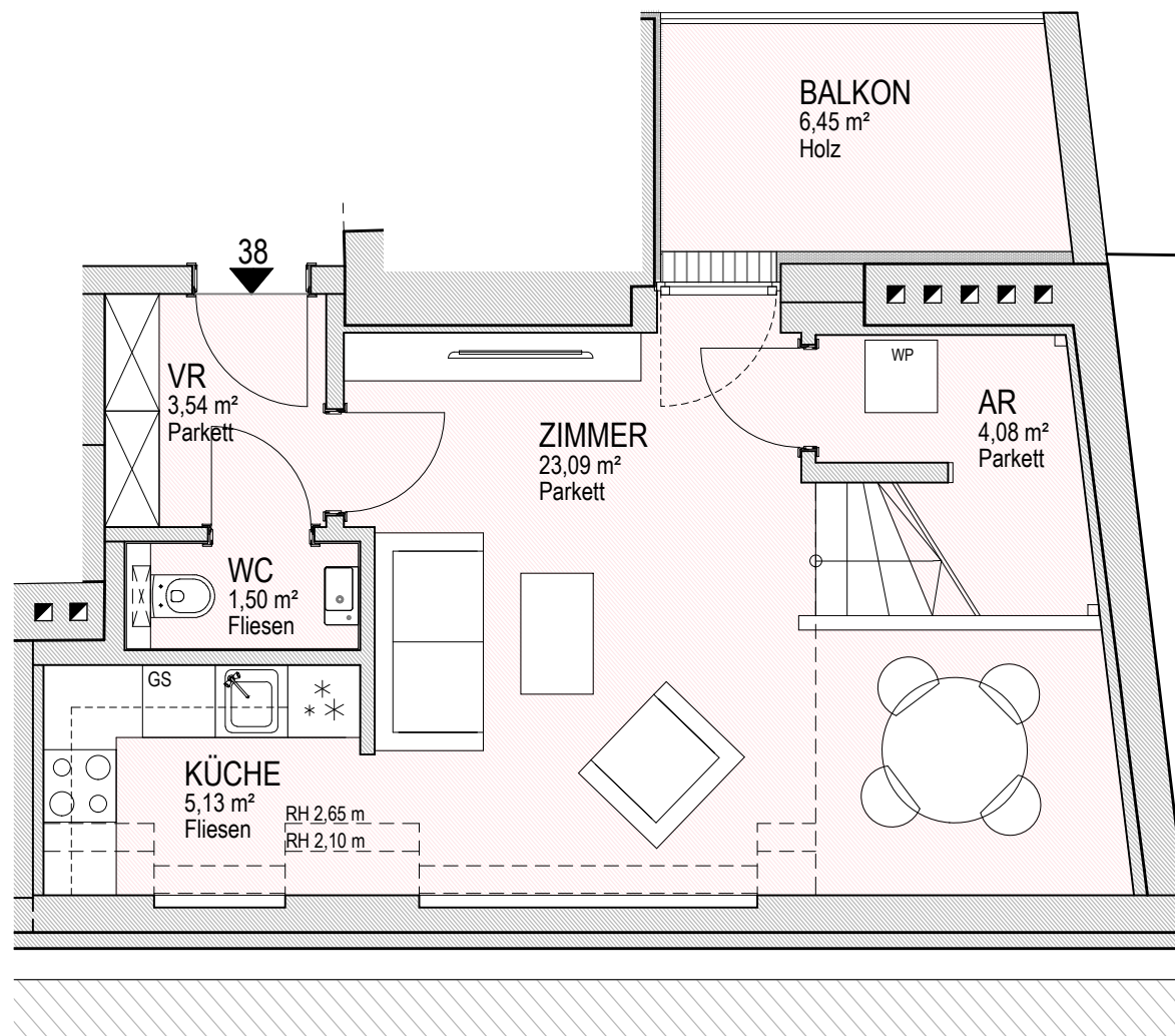
GRUNDRISS 1. DACHGESCHOSS
